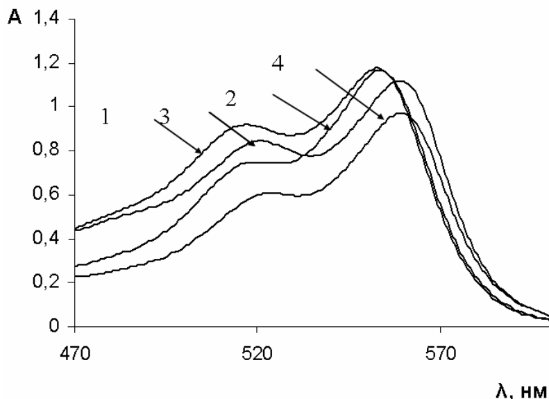
Рис. 3. Влияние Cu(II) на реакцию хлороксиминазо с Pd(II): 1 – комплекс Pd(II) ( 7,4 \cdot 10^{-5} M), 2 – комплекс Pd(II) в прис. равного количества Cu(II), 3 – комплекс Pd(II) в прис. 300-кратных количеств Cl - . 4 – комплекс Pd(II) в прис. равного количества Cu(II) и 300-кратных количеств хлорид-иона. Раствор сравнения – вода, l = 1 см
