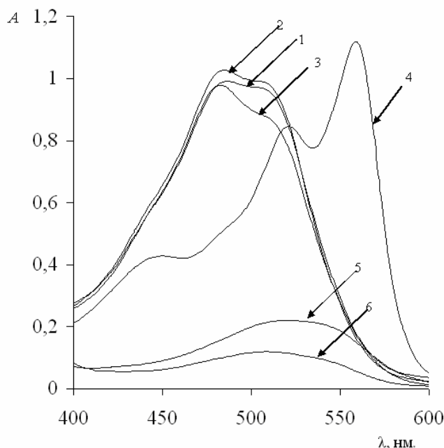
Рис. 1. Электронные спектры поглощения хлорксаминазо Ф (1) и его комплексов с Cr(III) (2), Ni(II) (3), Pd(II) (4), Cu(II) (5), Fe(III) (6) ( 7,4 \cdot 10^{-5} М растворы).
