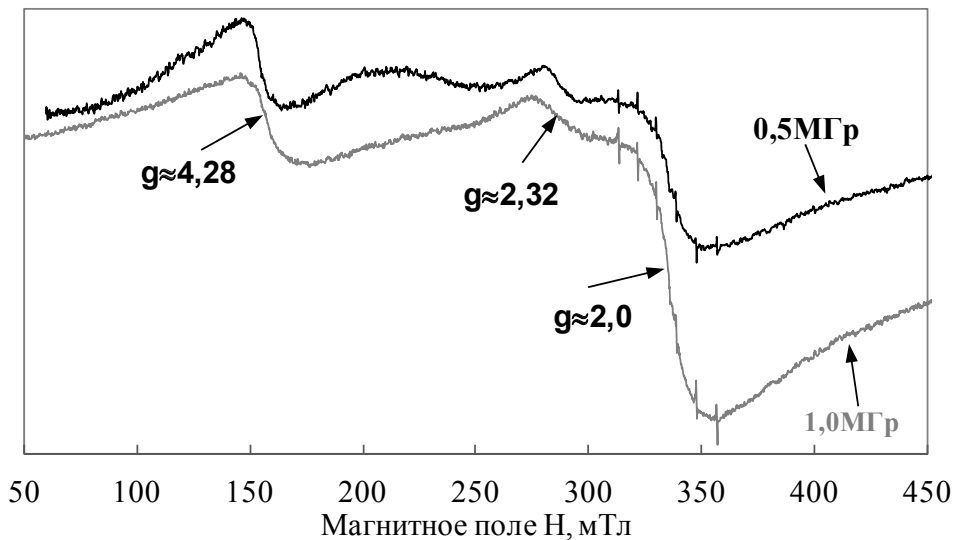
Рис. 4. Спектр ЭПР стекол 40 \text{ Na}_2\text{O}-15 \text{ Al}_2\text{O}_3-5 \text{ Fe}_2\text{O}_3-40 \text{ P}_2\text{O}_5 (мол.%), облученных электронами дозой 0,5 и 1,0 МГр.
