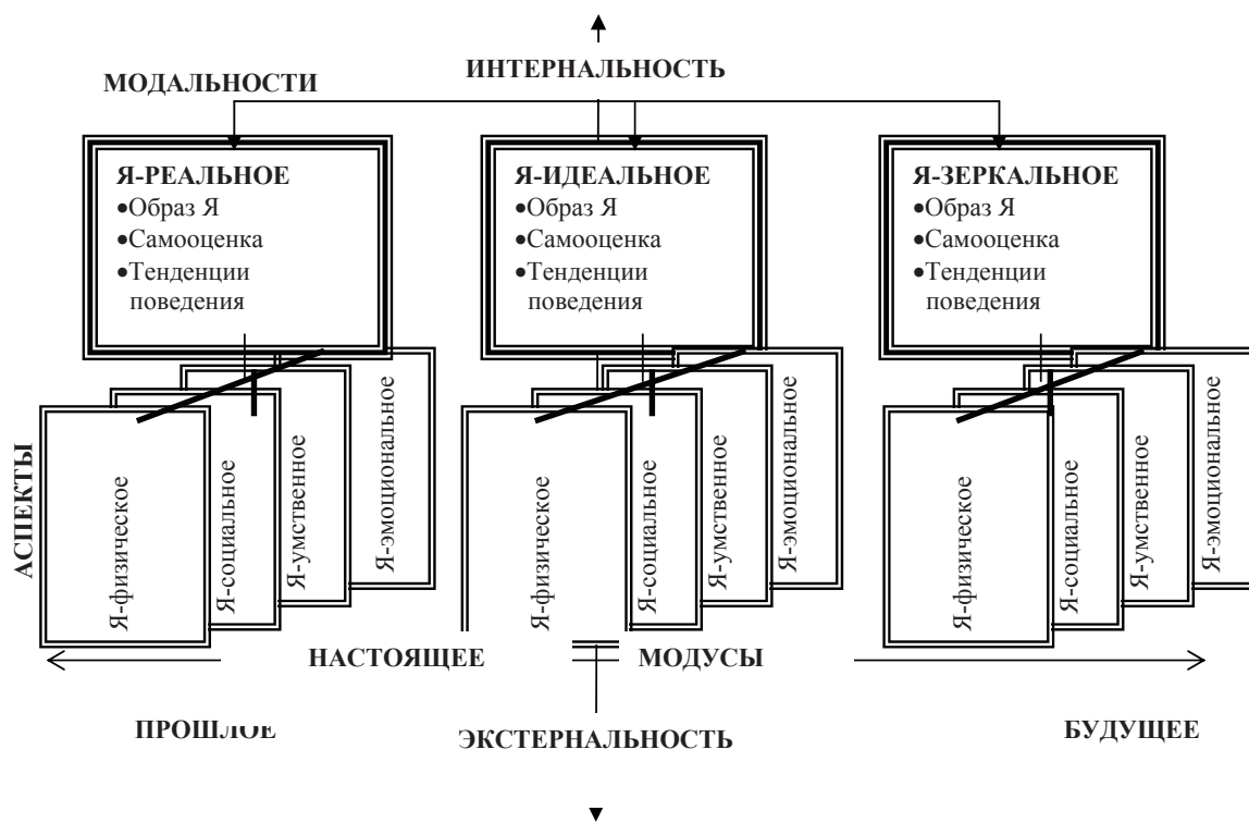
Рис. 1. Структура Я-концепции
